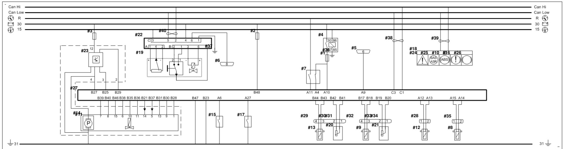
Abbildung 1: ABS > ABS-ASR Teves 20 (Gesamtdarstellung)
